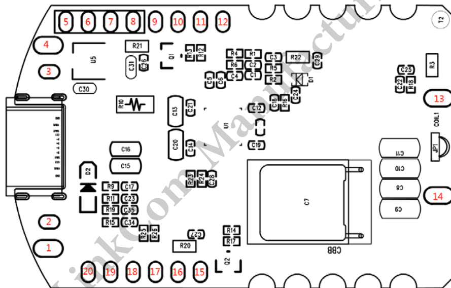
PCBA圖
