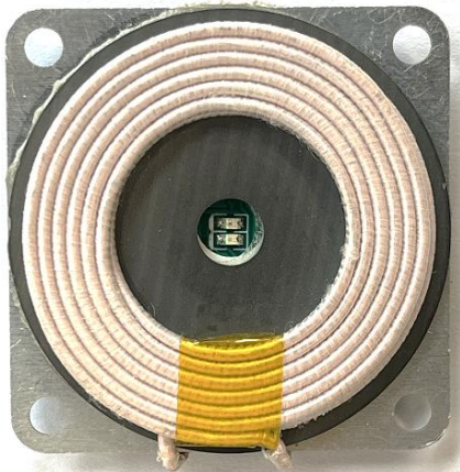
Module Front Side 模組前面
