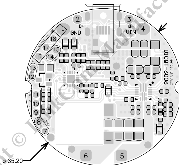
PCBA圖
